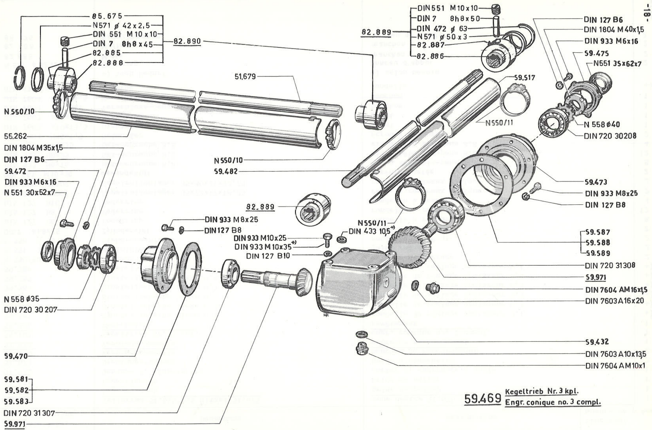
Kegeltrieb Nr.3
