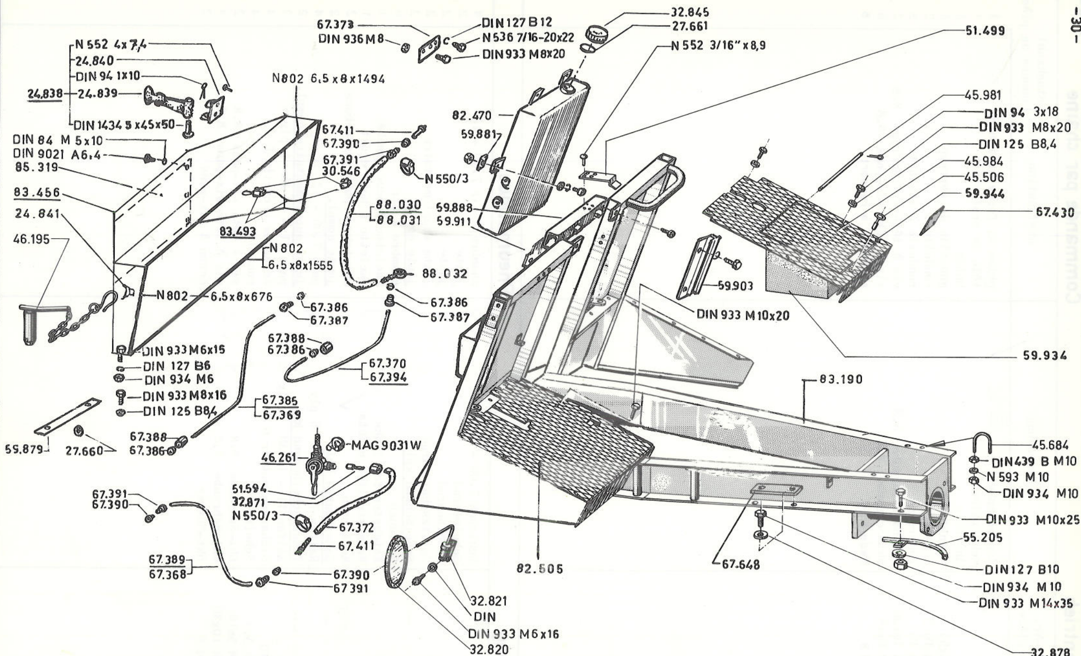
Frontaufbau, Kraftstoffanlage
