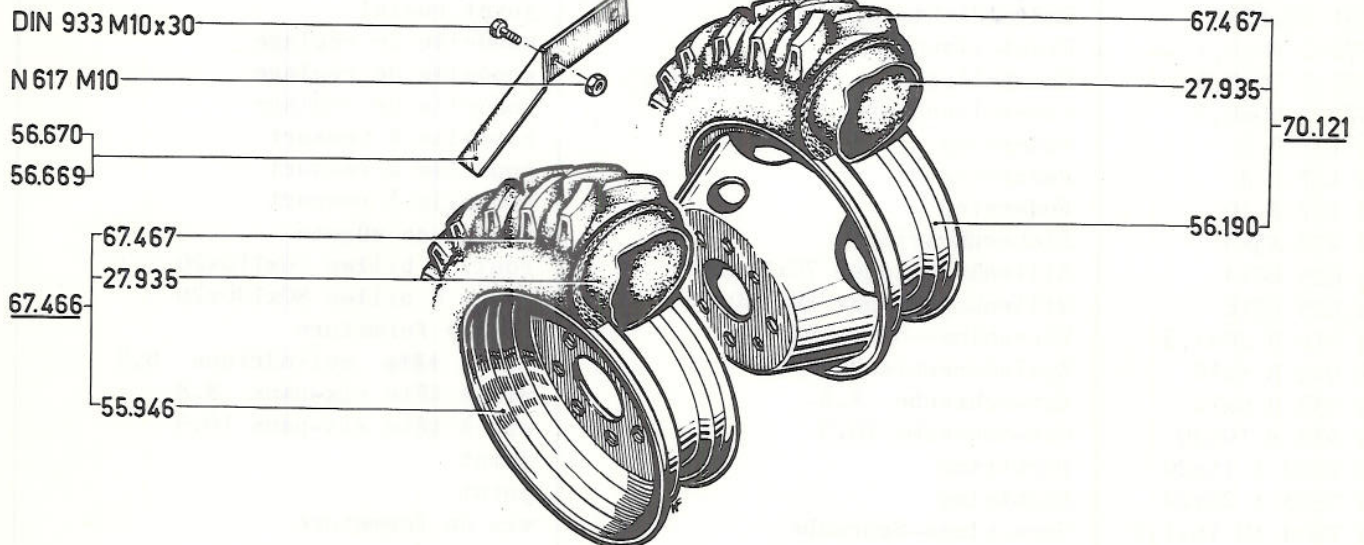
Bereifung
