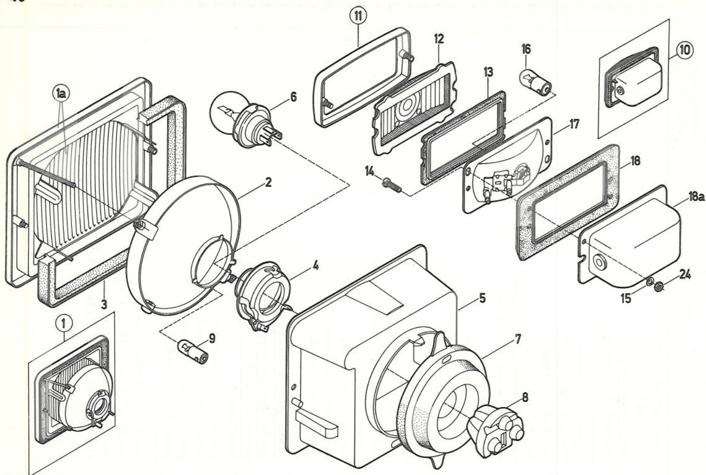
Blinkleuchte, Scheinwerfer
