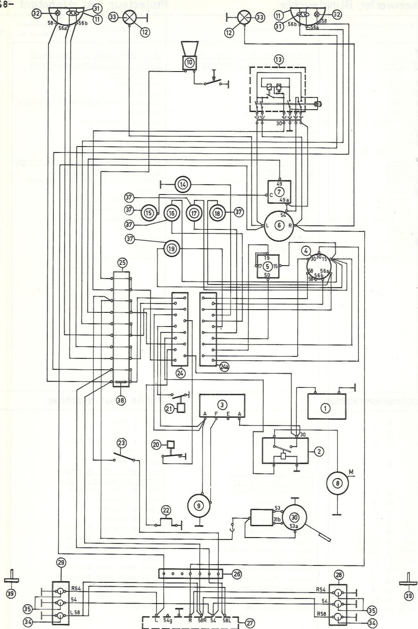
Schaltschema
