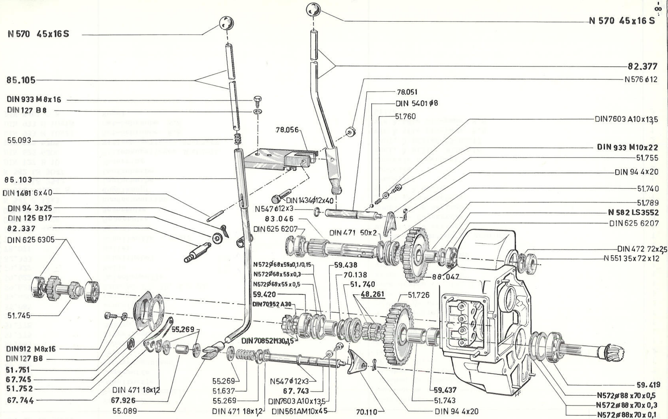
Retour-Ritzel-Zapfwelle
