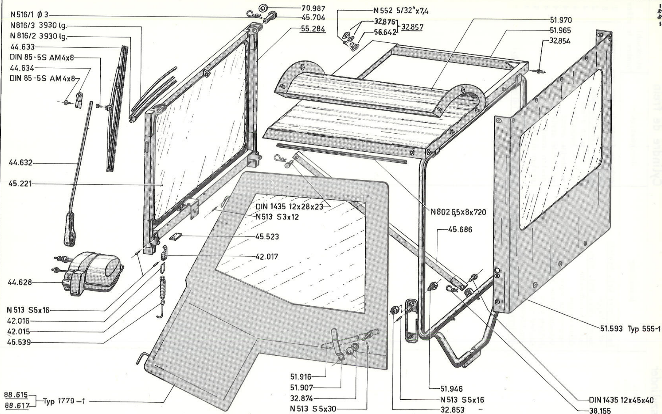
Verdeck-capote type 532-3 Rückwand — panneau arrière type 555-1 Türen — portes type 1779-1
